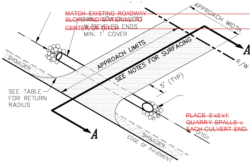
PLAN N.T.S.
